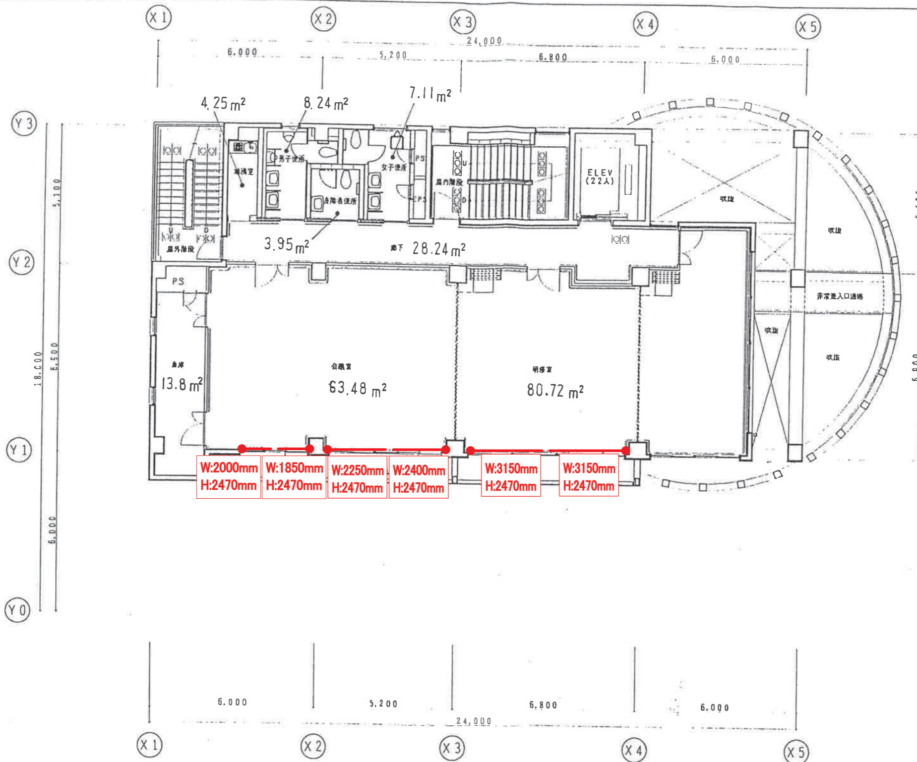
5階平面図
