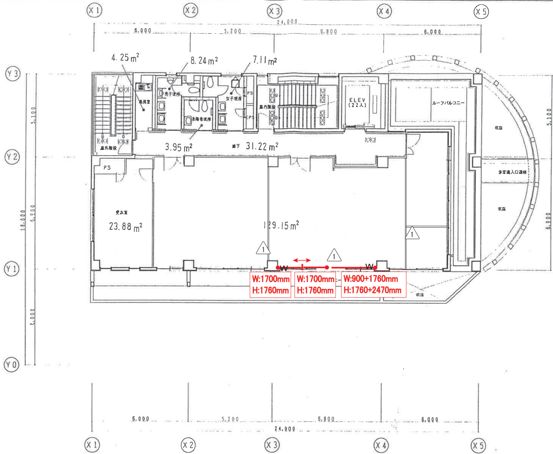
4階平面図
