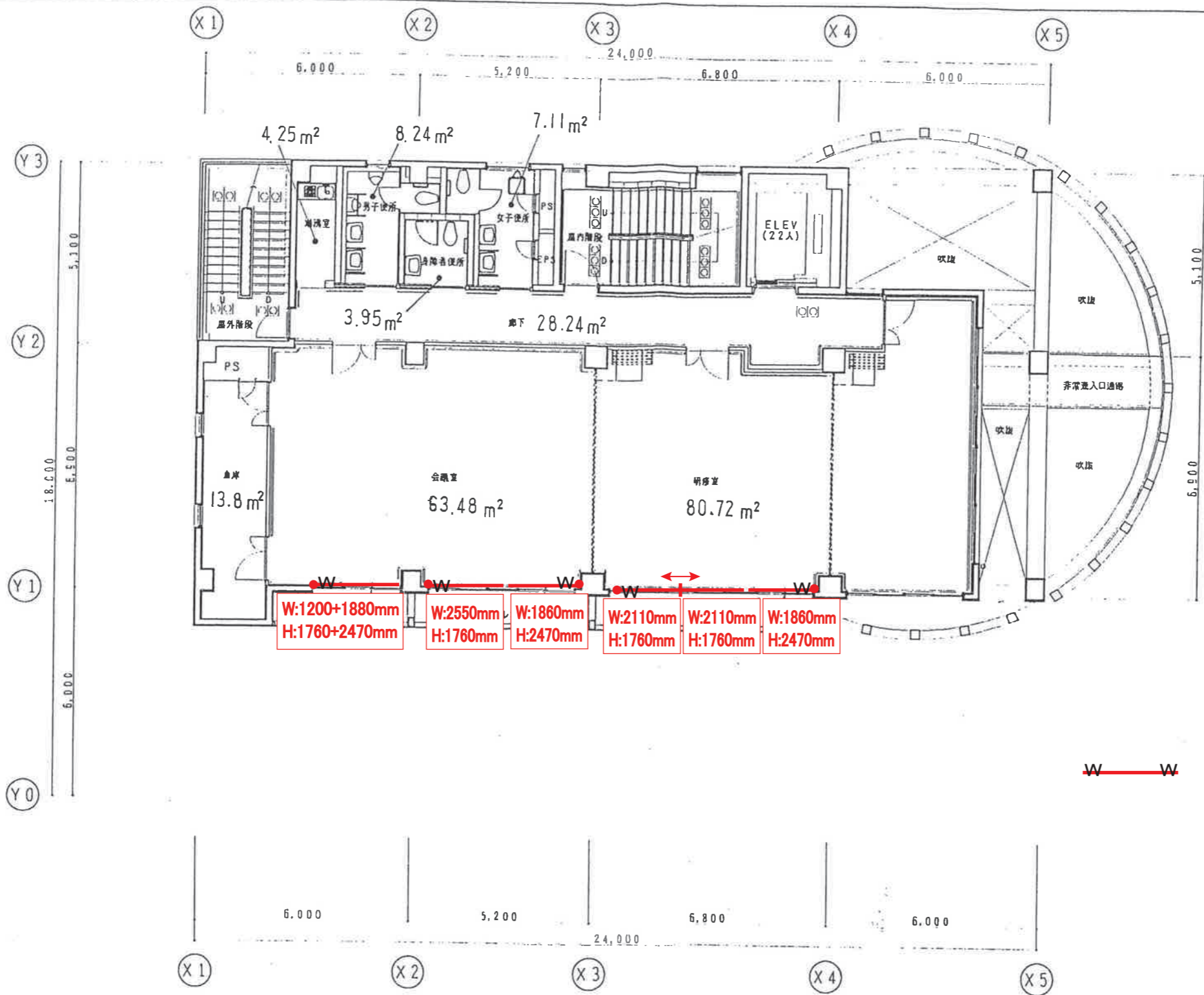
5階平面図
